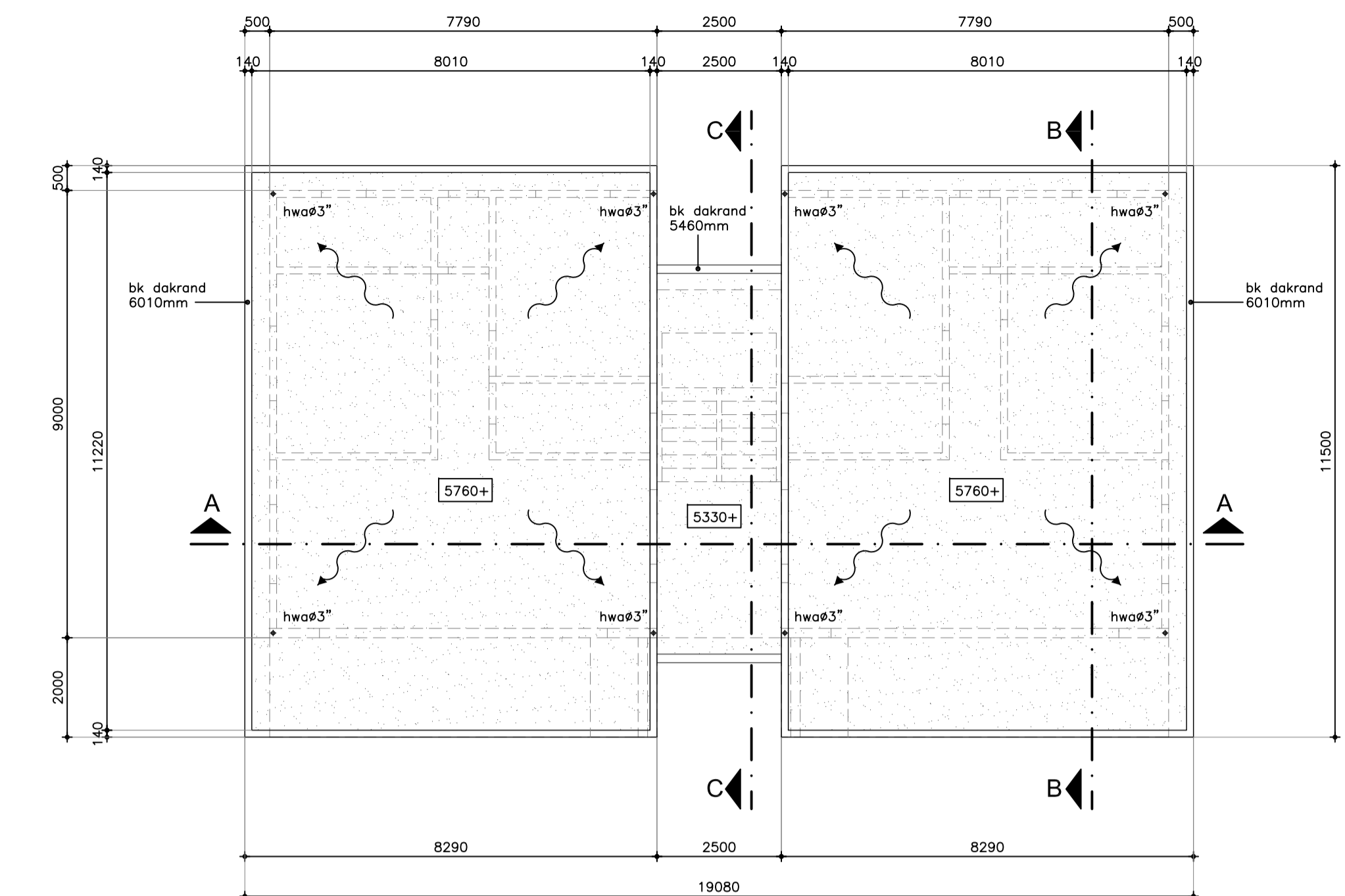
DAKPLAN APPARTEMENT TYPE B
