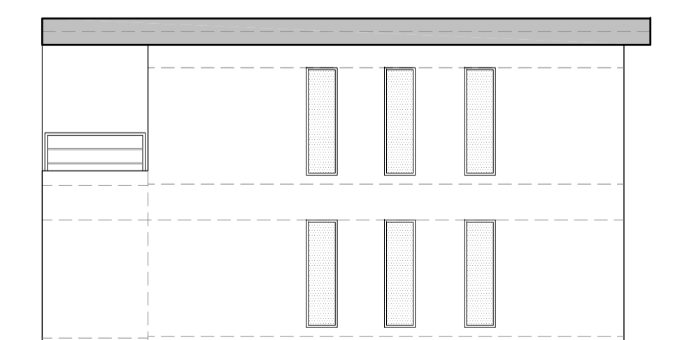
RECHTER ZIJGEVEL APPARTEMENT TYPE B
